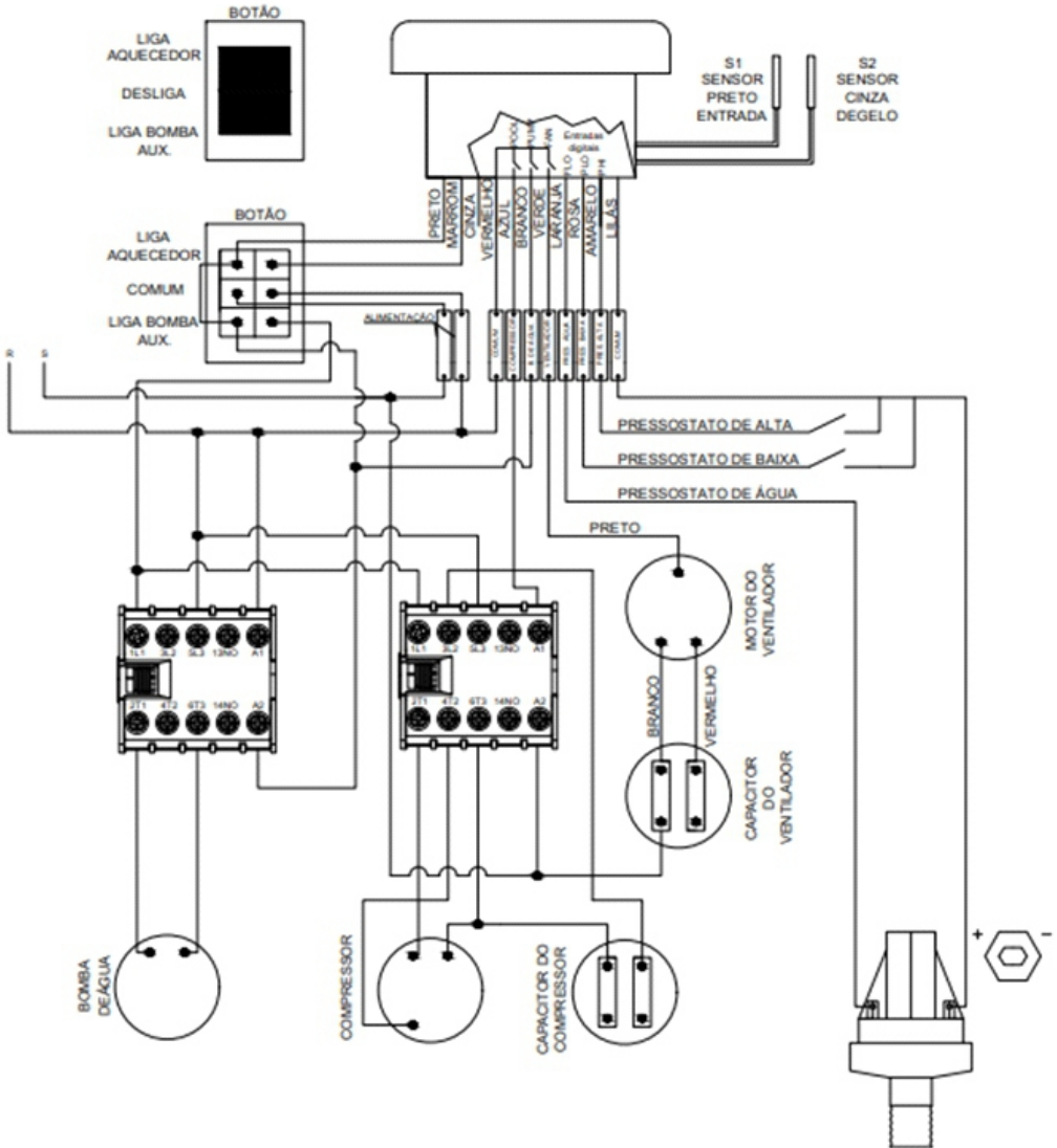
ESQUEMA ELÉTRICO MONOFASICO-220V - ID15 - HOTSPA
