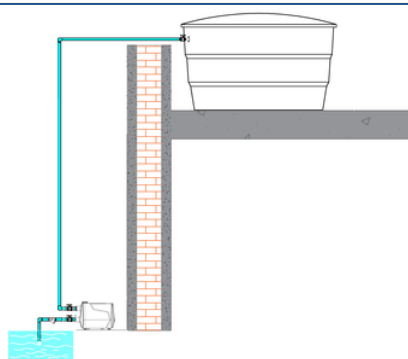
Recalque para reservatório superior
